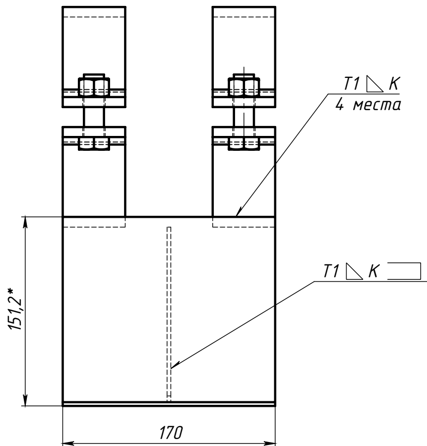
Поз.3 (Ребро среднее)
