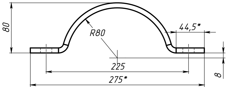
Поз.4 (Полухомут) развертка
