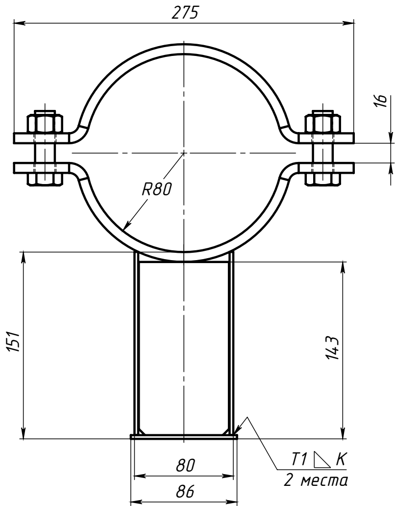
Поз.4 (Полухомут)
