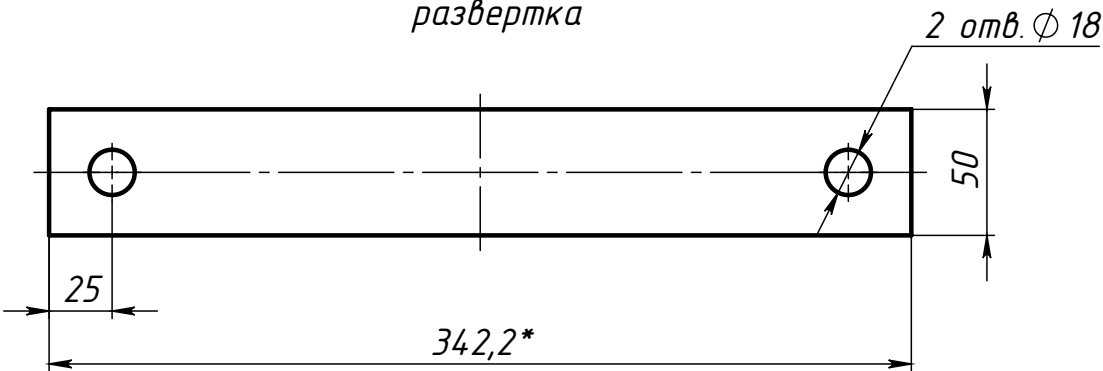
Поз.4 (Полухомут) развертка
